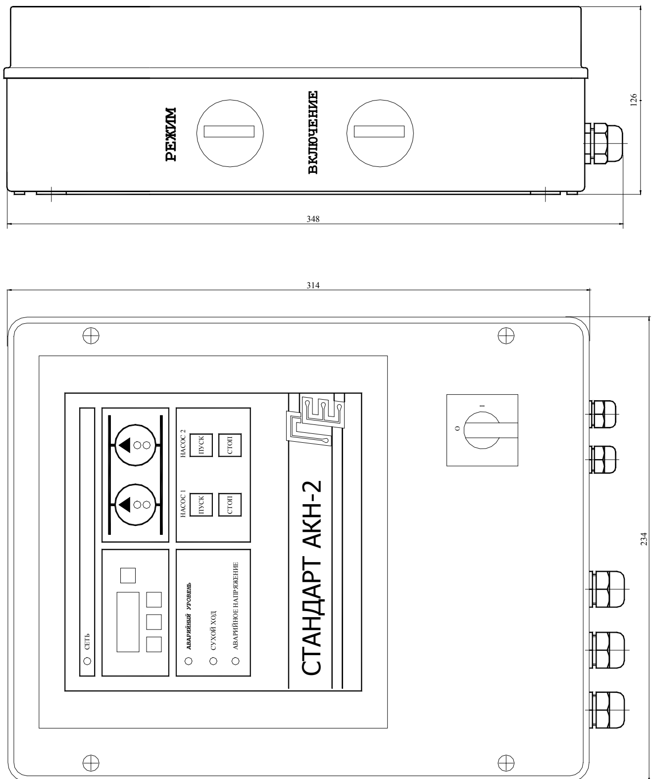
Рисунок А.1 – Общий вид устройства СТАНДАРТ АКН-2Д
