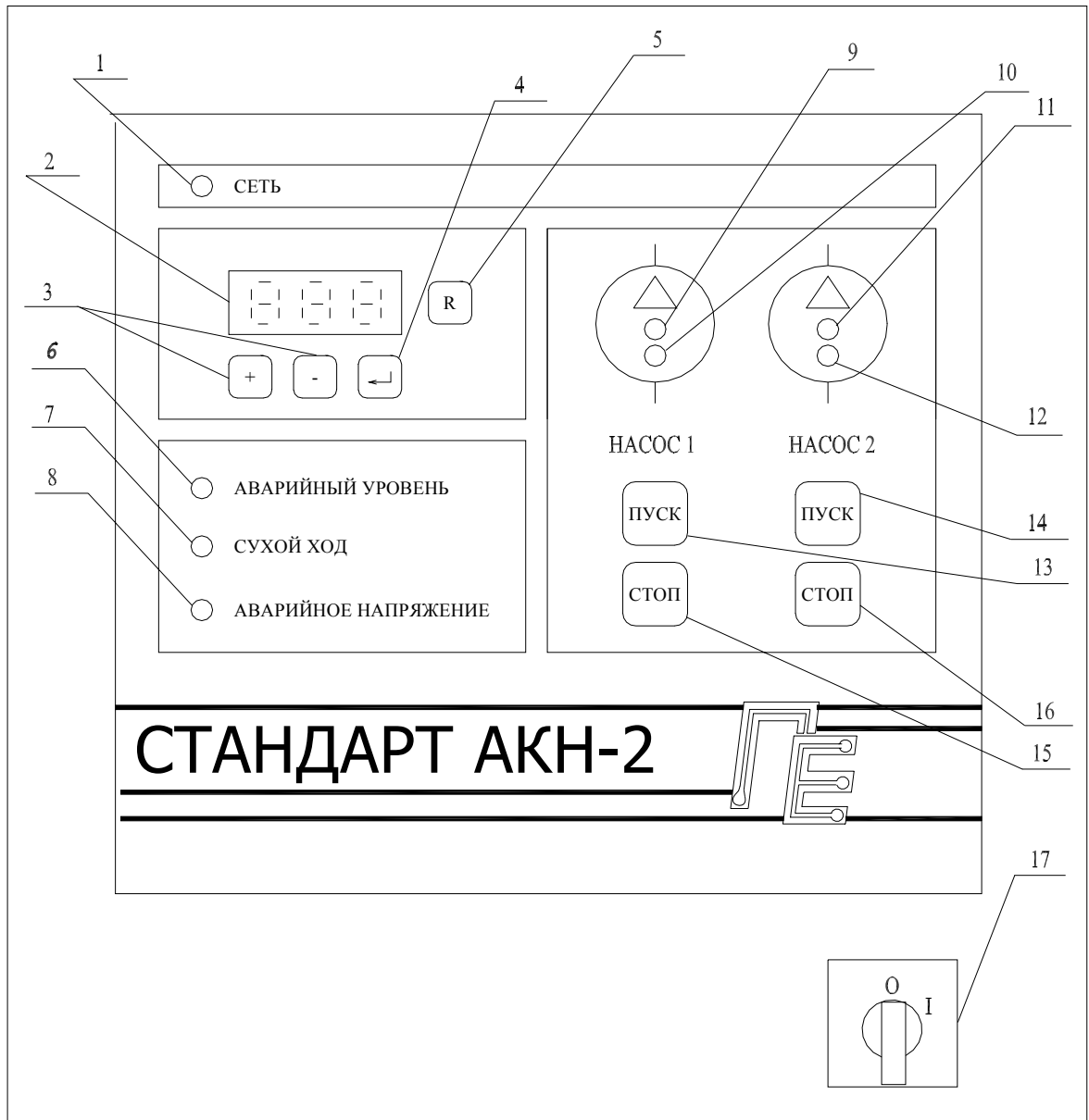
Рисунок 1 – Лицевая панель устройства СТАНДАРТ АКН-2Д
